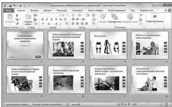
Рис. 16. Готовая презентация
