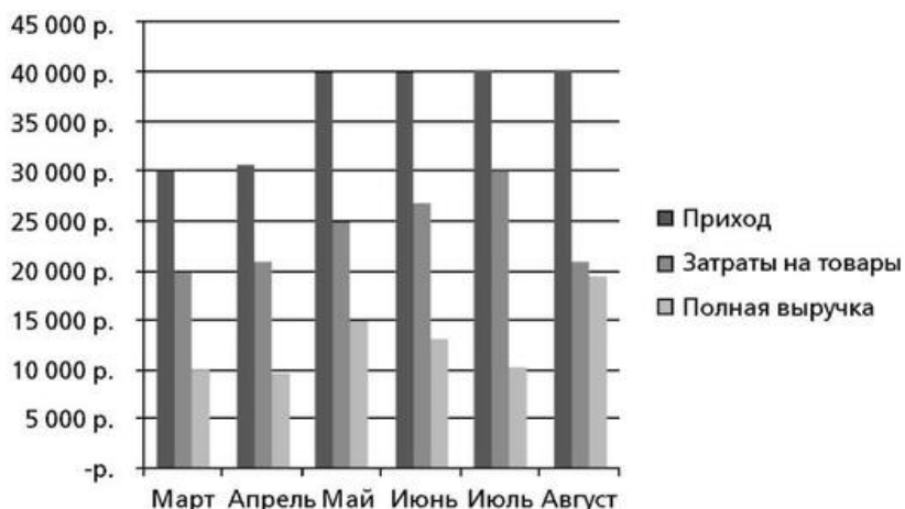
Рис.8 Построенная гистограмма
