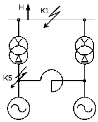
Рис. 4.2. Схема станции № 1
