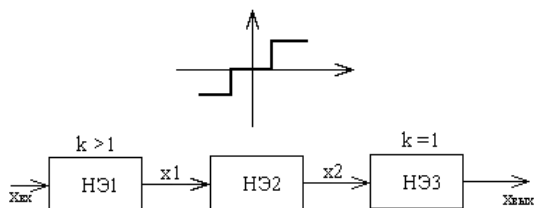
Рис. 42. Схема статической характеристики НЭ
