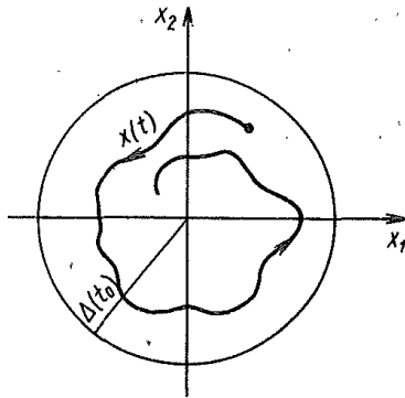
Рис. 33. Фазовый портрет асимптотически устойчивой траектории
