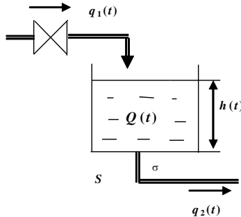
Рис. 1. Схема гидравлического объекта-резервуара
