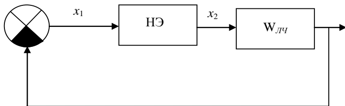
Рис. 40. Каноническая структурная схема НСАУ
