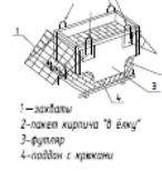
Подача пакета кирпича захватом-фуллером
