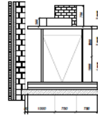
КЛАДКА ТРЕТЬЕГО ЯРУСА СТЕН
