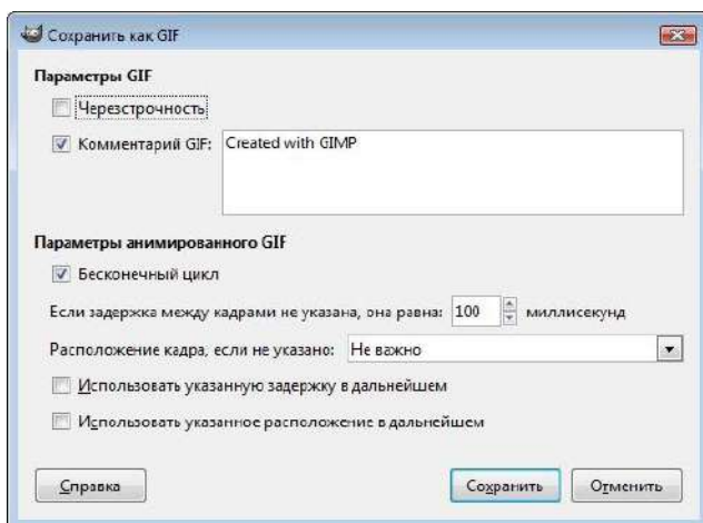
Рис. 6. Сохранение GIF
