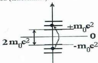
Рис. 7.7. Переход электрона с отрицательного уровня энергии на положительный (энергия перехода h\nu \geq m_0c^2 )
